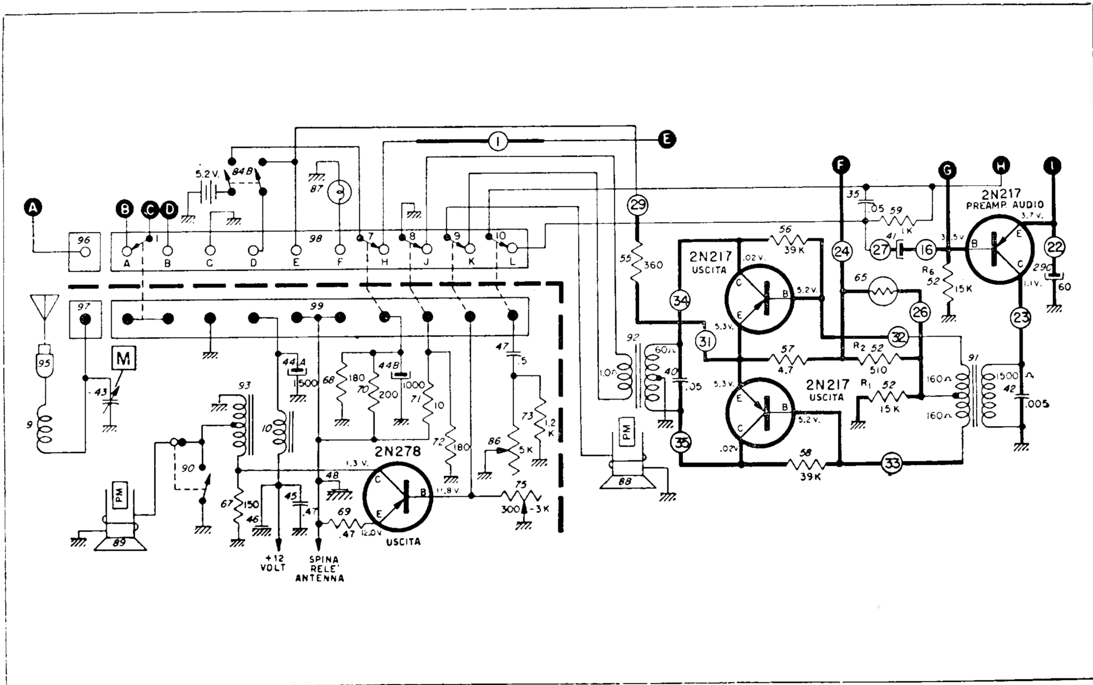
Fig. 9-2. - Radiorecettore totalmente a transistori per auto, mod. 98837 (Pontiac) della Delco.
